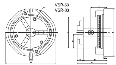
VSR-63 + VSC-6A 3JAW CHUCK VSR-83 + VSC-8A 3JAW CHUCK
