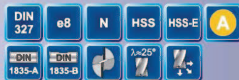
DIN 327-B K
