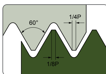
UNC, UNF, UNEF ANSI B1.1-1982
